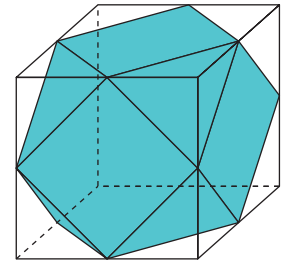
CUBO - CUBOCTAEDRO
